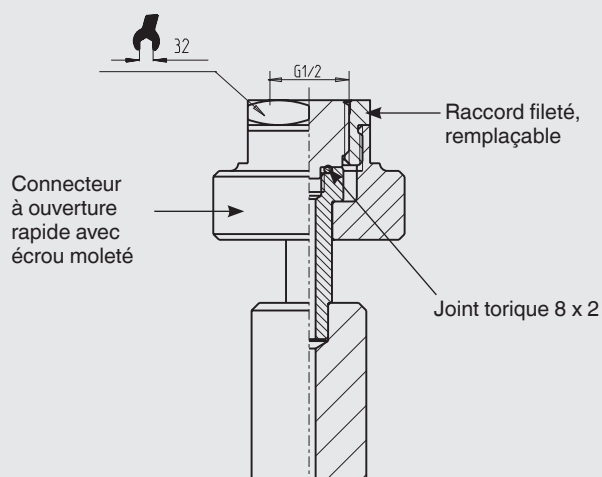
Raccord pour l'instrument sous test
